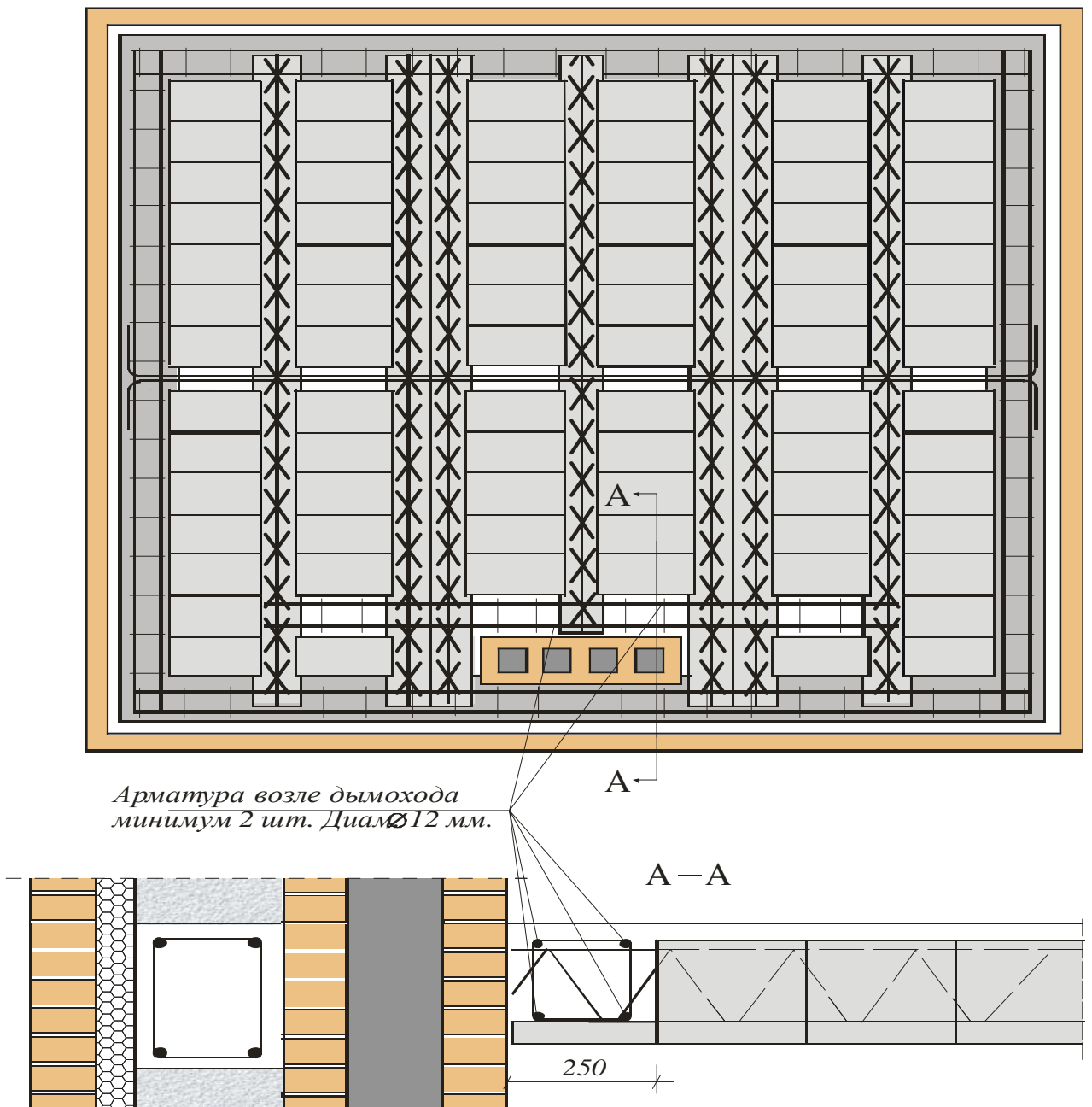
Рис. 25 Укладка балок и пустотелых блоков возле дымохода.
