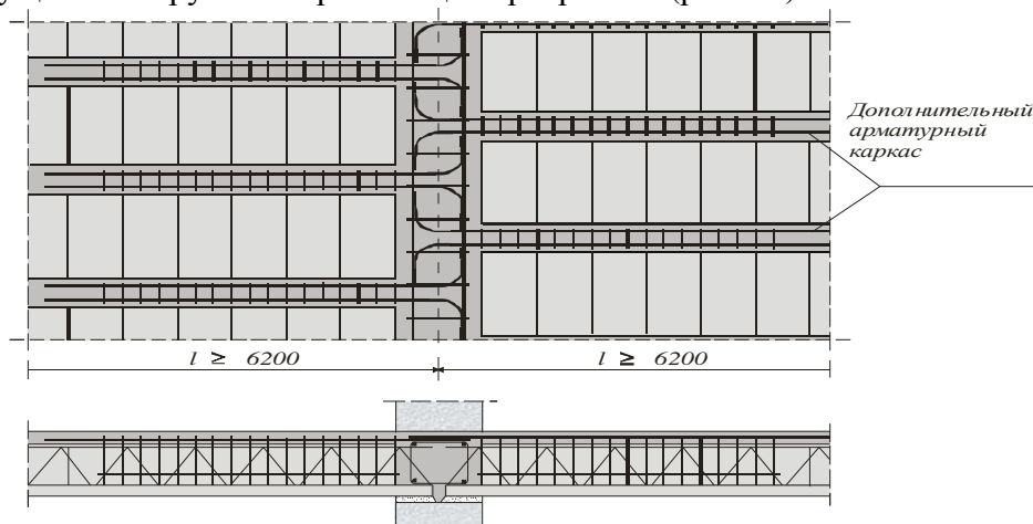
Рис. 11 Расположение дополнительного арматурного каркаса перекрытия «TERIVA NOVA», используемого в зоне опоры балок перекрытия «TERIVA NOVA» на стену, находящиеся на разных уровнях.
