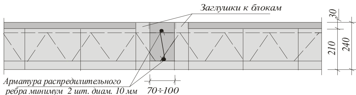
Рис. 22 Поперечное сечение распределительного ребра в перекрытии «Teriva-I», с применением заглушек для блоков.
