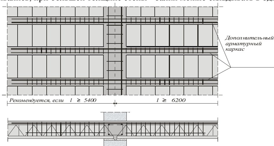
Рис. 12 Расположение дополнительного арматурного каркаса перекрытия «TERIVA NOVA», используемого в зоне опоры балок перекрытия «TERIVA NOVA» на стену, находящиеся на одном уровне.
