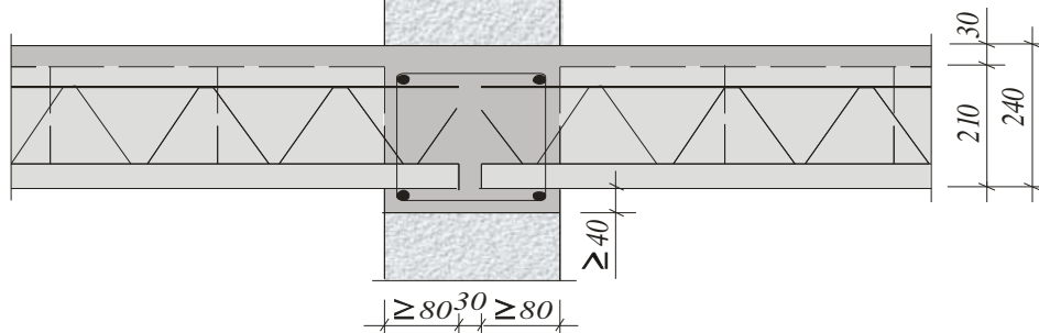
Рис. 19 Венец, связывающий перекрытие на внутренней несущей стене, приподнятый на 4 см.
