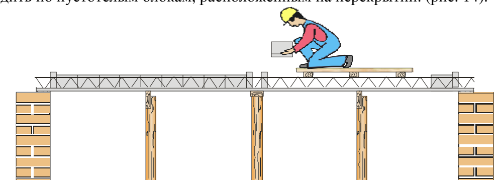
Рис. 14 Монтаж пустотелых блоков перекрытий с рабочих помостов, находящихся с верху и расположенных перпендикулярно балкам перекрытия
