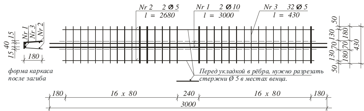
Рис. 6 Дополнительный арматурный каркас, используемый в зоне опоры балок перекрытия «TERIVA NOVA» на стену, находящиеся на одном уровне.
