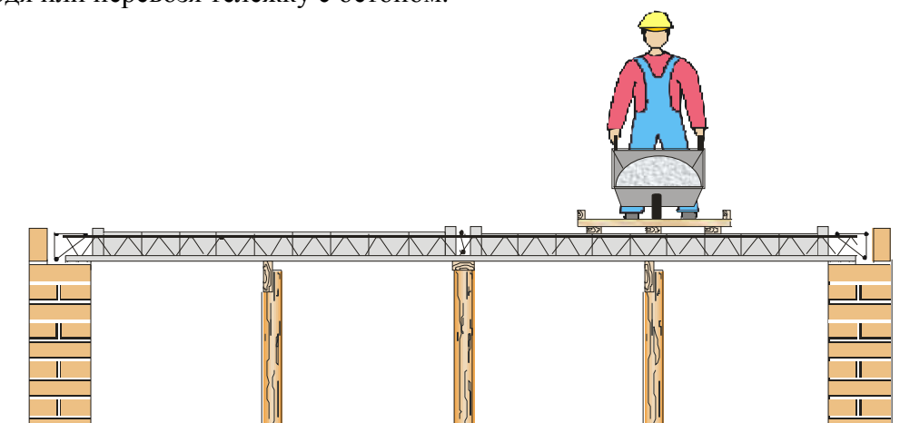
Рис. 15 Бетонирование перекрытия с рабочих помостов, расположенных перпендикулярно балкам перекрытия.
