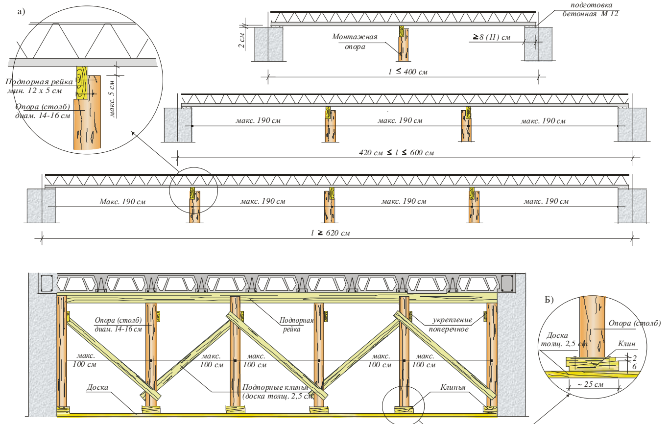
Рис. 3 Способ подпираания балок Teriva на период монтажа и бетонирования перекрытия.
